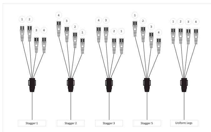
Beispiele für Harness-Stufenmuster | Foto ZA4253
