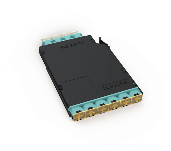
EDGE 4x6 Konvertierungsmodul | Foto REN7071
