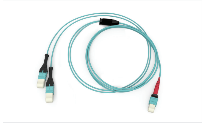
EDGE 24-Faser “Y” Harness | Foto REN7941
