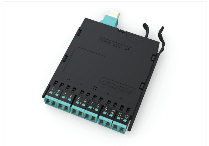
EDGE Modul | Foto REN6521
