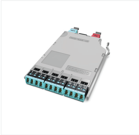
MTP zu LC Duplex Multimode TAP Modul | Foto REN3557
