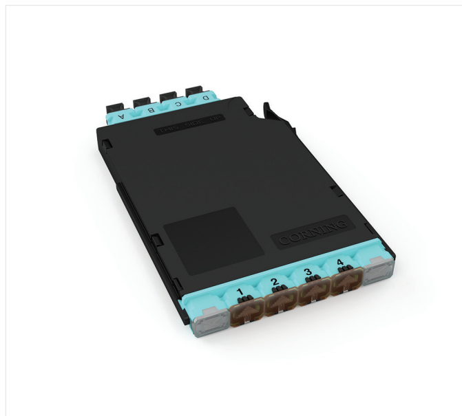
EDGE Multimode Mesh Modul | Foto REN890
