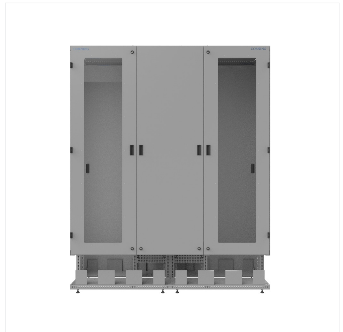
EDGE™ Doppel-Verteilerschrank mit rückseitigem Zugriff | Foto REN9402
